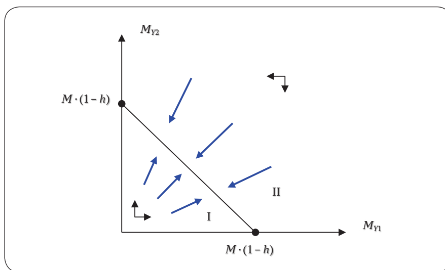
Рис. 4. Фазовый портрет системы (23) – (24) при условии h_i = h
